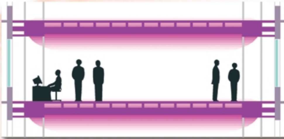
Snittegning gjennom hovedkontoret til GSW i Berlin, der eksponert betong i himlingen akkumulerer overskuddsvarme på dagtid (venstre). Overskuddsvarmen ventileres bort nattestid ved naturlig kryssventilasjon (høyre).
